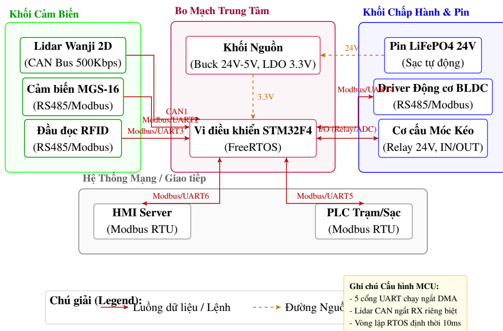
Hình 3.2 Sơ đồ khối kết nối hệ thống phần cứng xe tự hành AGV B400.
